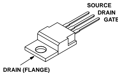
JEDEC TO-220AB
